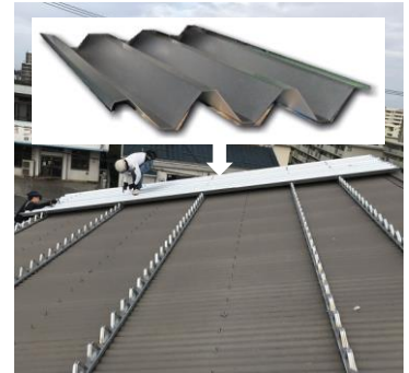
ルーフ二重張り施工
