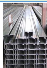
C型鋼 2.3×60×30
